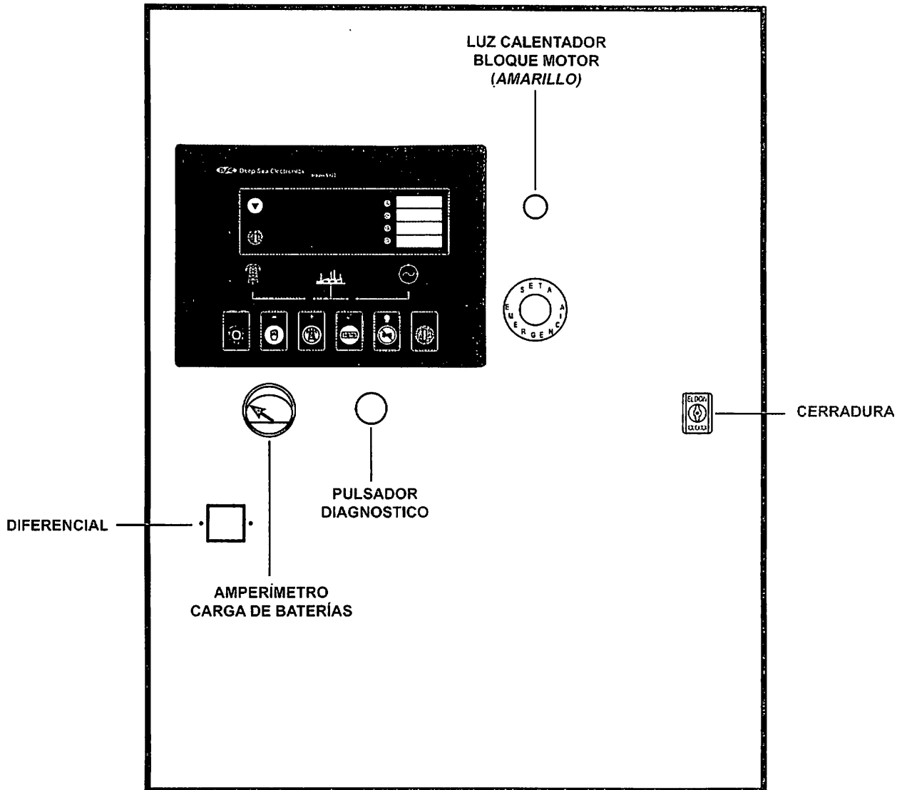
Imagen 6 - CUADRO DE CONTROL DE PLACA DE CONTROL DEEPSEA
