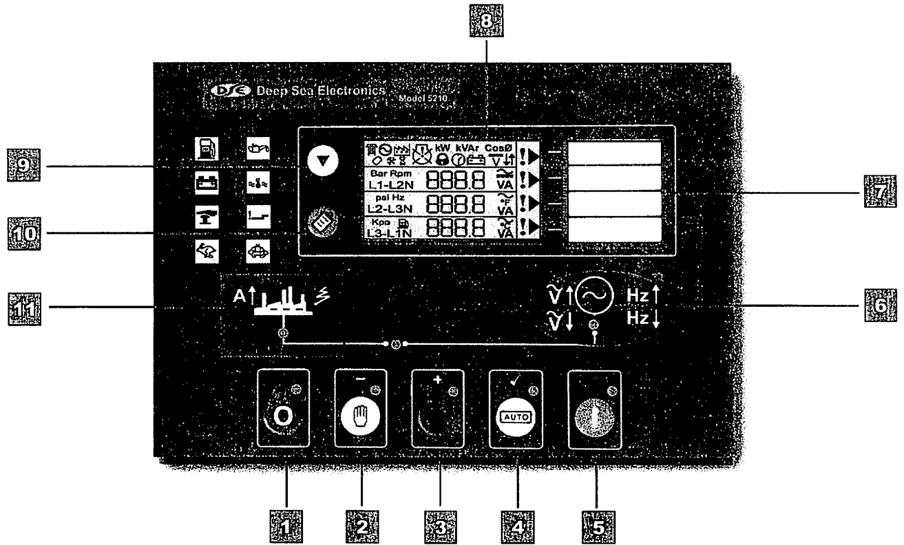
Imagen 11 - PLACA DE CONTROL DEEP SEA 5210
