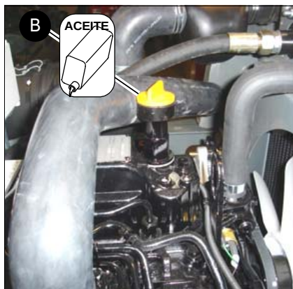
Fig. 28: Añadir aceite motor
