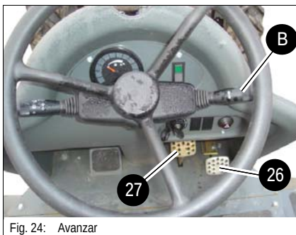
Fig. 24: Avanzar
