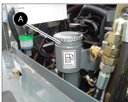
Fig. 23: Tubuladura de llenado de combustible
