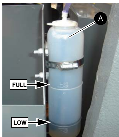
Fig. 29: Depósito de expansión del líquido refrigerante
