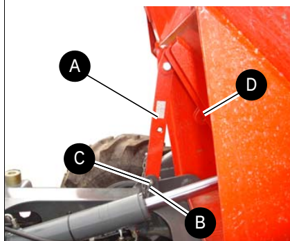
Fig. 21: Soporte de mantenimiento volquete frontal
