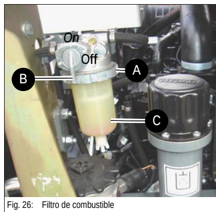
Fig. 26: Filtro de combustible
