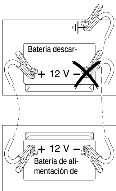
Fig. 23: Ayuda de arranque con cables de arranque
