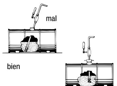
Fig. 24: Repostar combustible desde un barril
