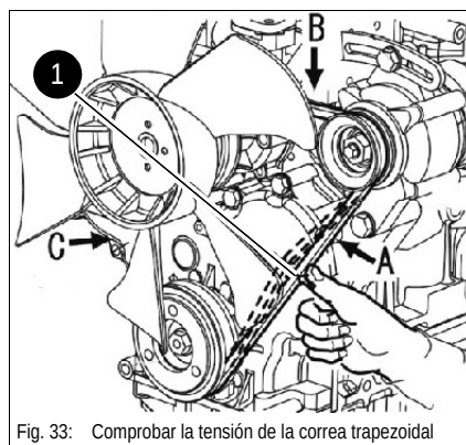
Fig. 33: Comprobar la tensión de la correa trapezoidal
