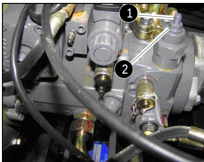
Fig. 41: Abrir circuito de alta presión
