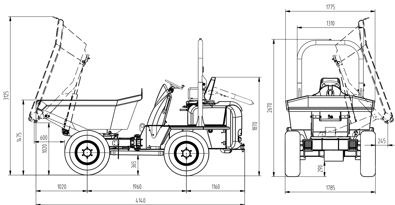
Fig. 45: Dimensiones del vehículo (modelo 3001S)
