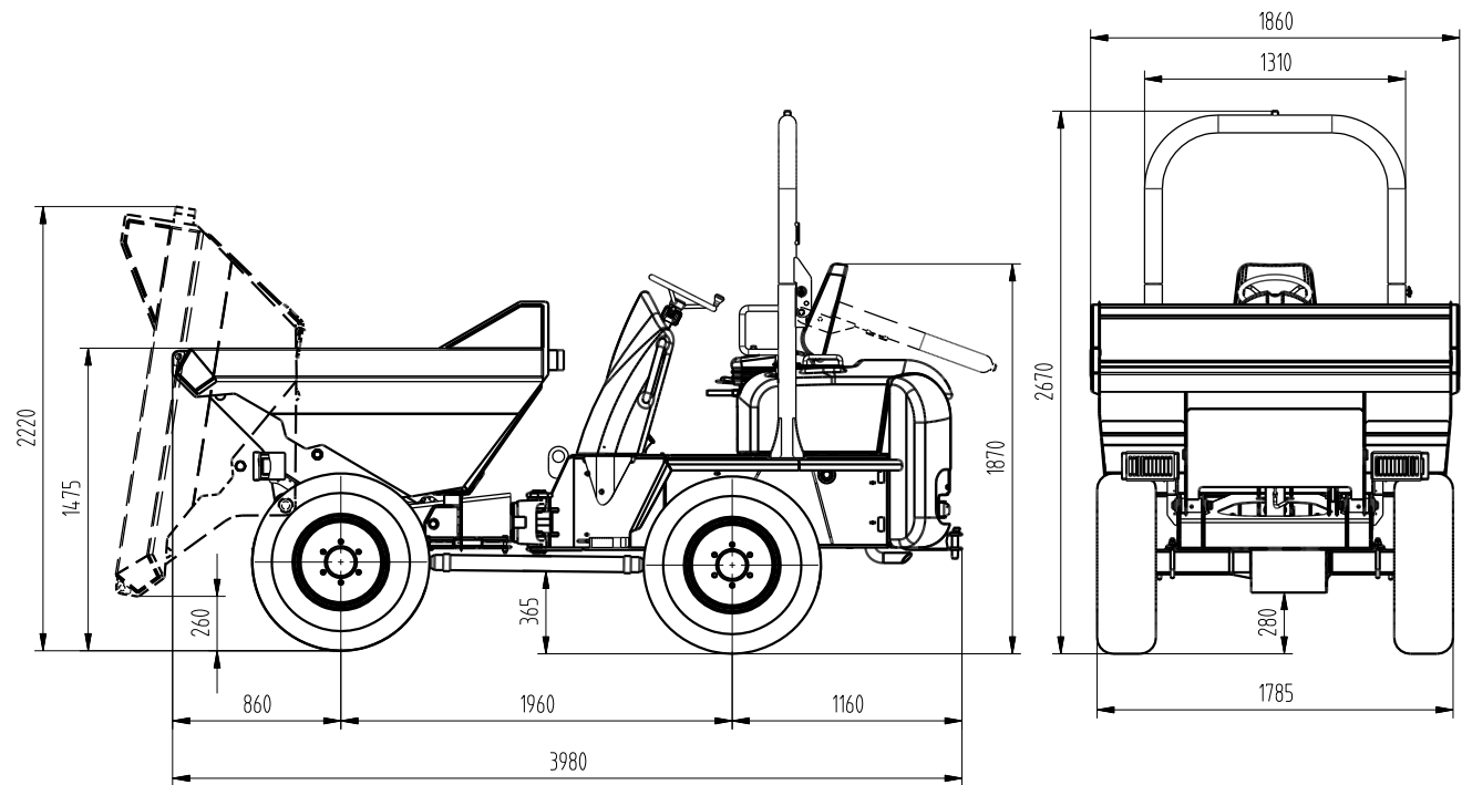
Fig. 44: Dimensiones del vehículo (modelo 3001 F)
