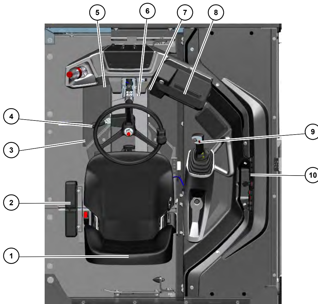
Fig. 84 Vista general elementos de mando
