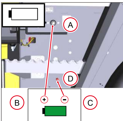
Fig. 126: Sistema auxiliar para la puesta en marcha
