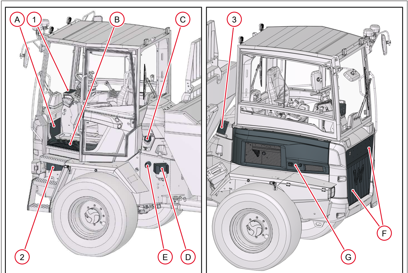
Fig. 200: Accesos de mantenimiento DV60/DV90/DV100
