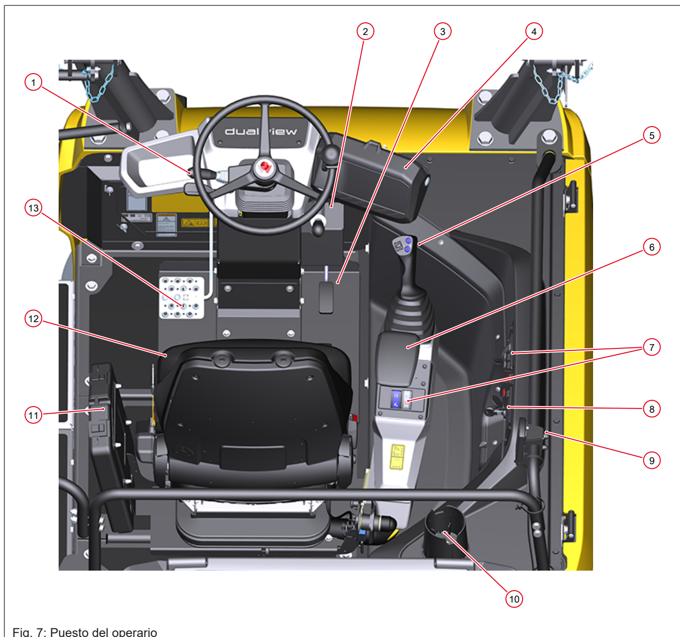
Fig. 7: Puesto del operario
