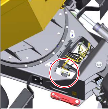
Fig. 231: Depósito de agua limpiaparabrisas volquete giratorio
