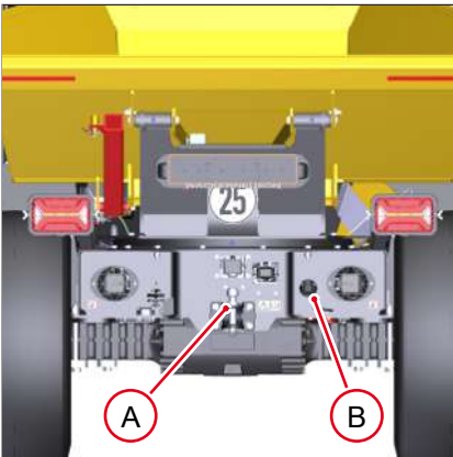
Fig. 155: Posición del dispositivo de acoplamiento
