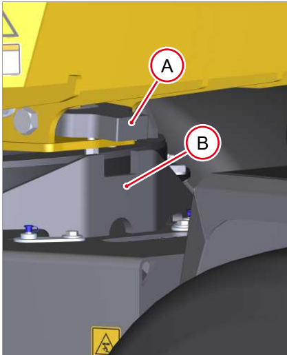
Fig. 181: Desbloquear el volquete
