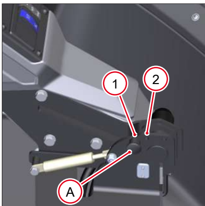
Fig. 93: Ajuste del soporte de la palanca de mando
