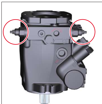
Fig. 185: Válvulas limitadoras de presión
