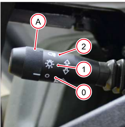
Fig. 161: Palanca multifunción
