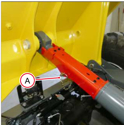
Fig. 236: Apoyo de mantenimiento montado
