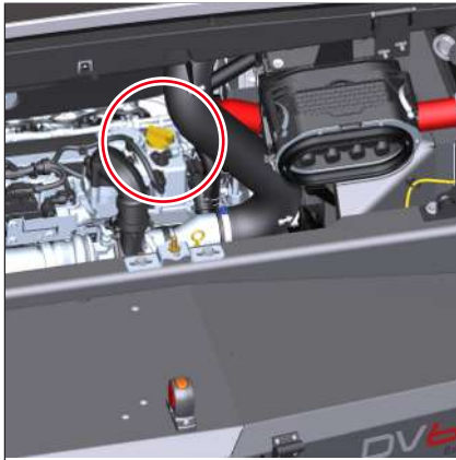
Fig. 221: Abertura de llenado para el aceite del motor
