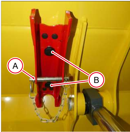
Fig. 235: Sujeción al volquete
