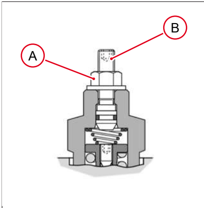
Fig. 187: Válvulas limitadoras de presión
