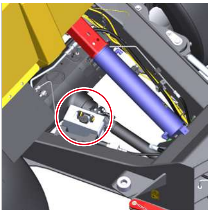
Fig. 230: Depósito de agua limpiaparabrisas volquete delantero
