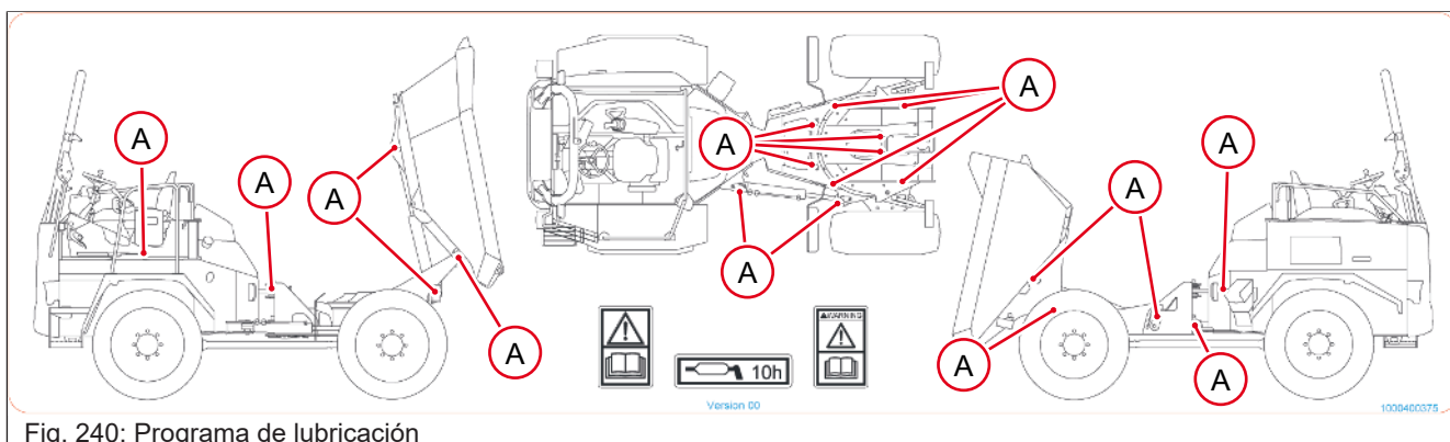
Fig. 240: Programa de lubricación
