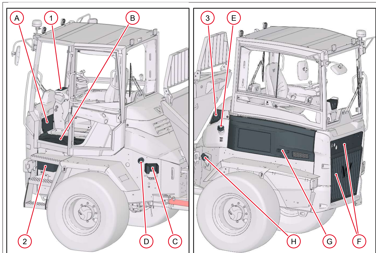
Fig. 201: Accesos de mantenimiento DV60 power/DV90 power
