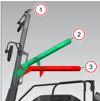
Fig. 105: Posiciones barra antivuelco
