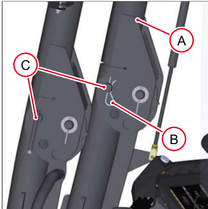
Fig. 103: Barra antivuelco: pasador y perno
