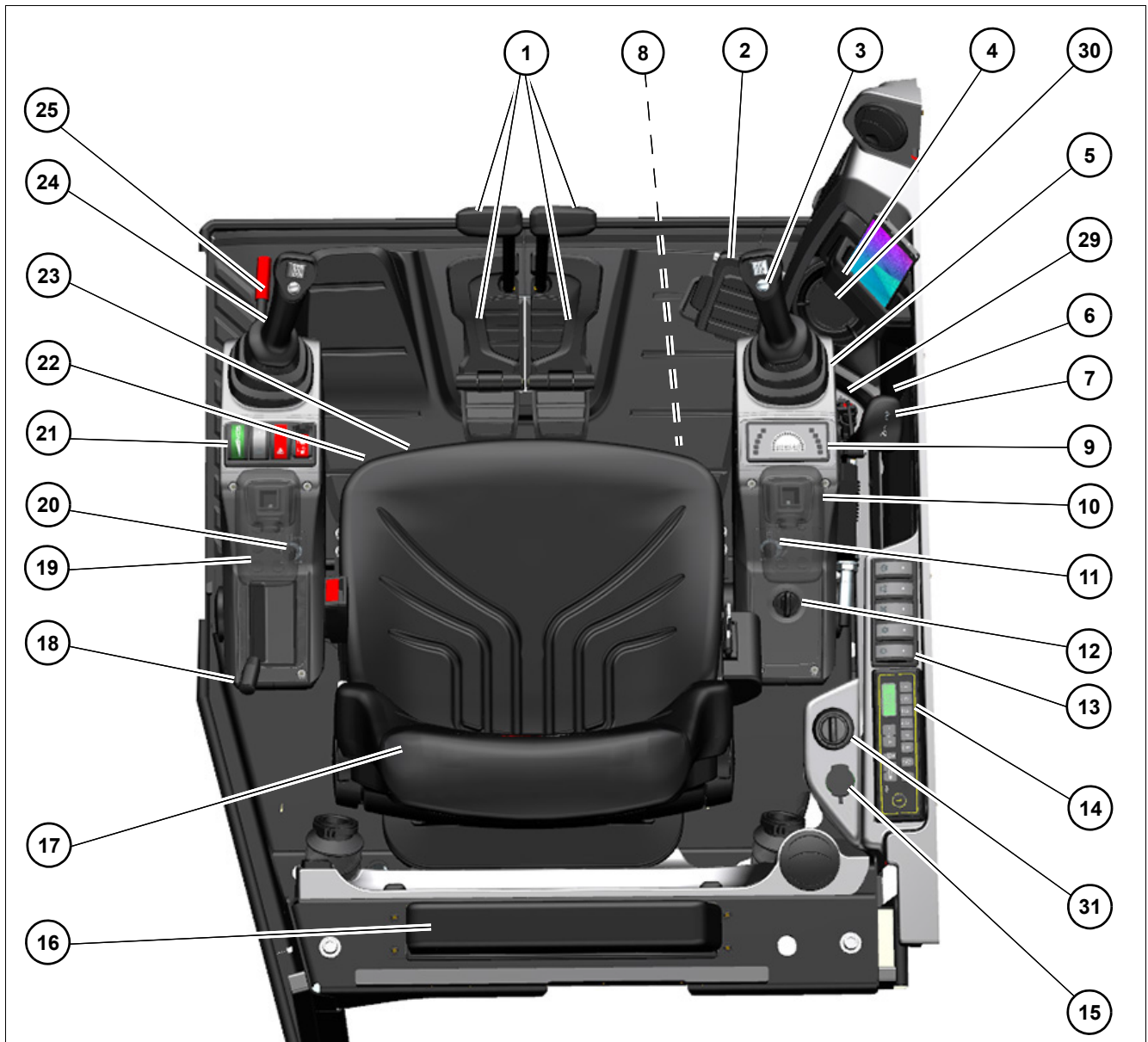
Fig.111 Vista general de los elementos de mando (3TNV88)
