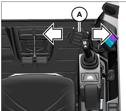
Fig.165 Bascular el brazo saliente
